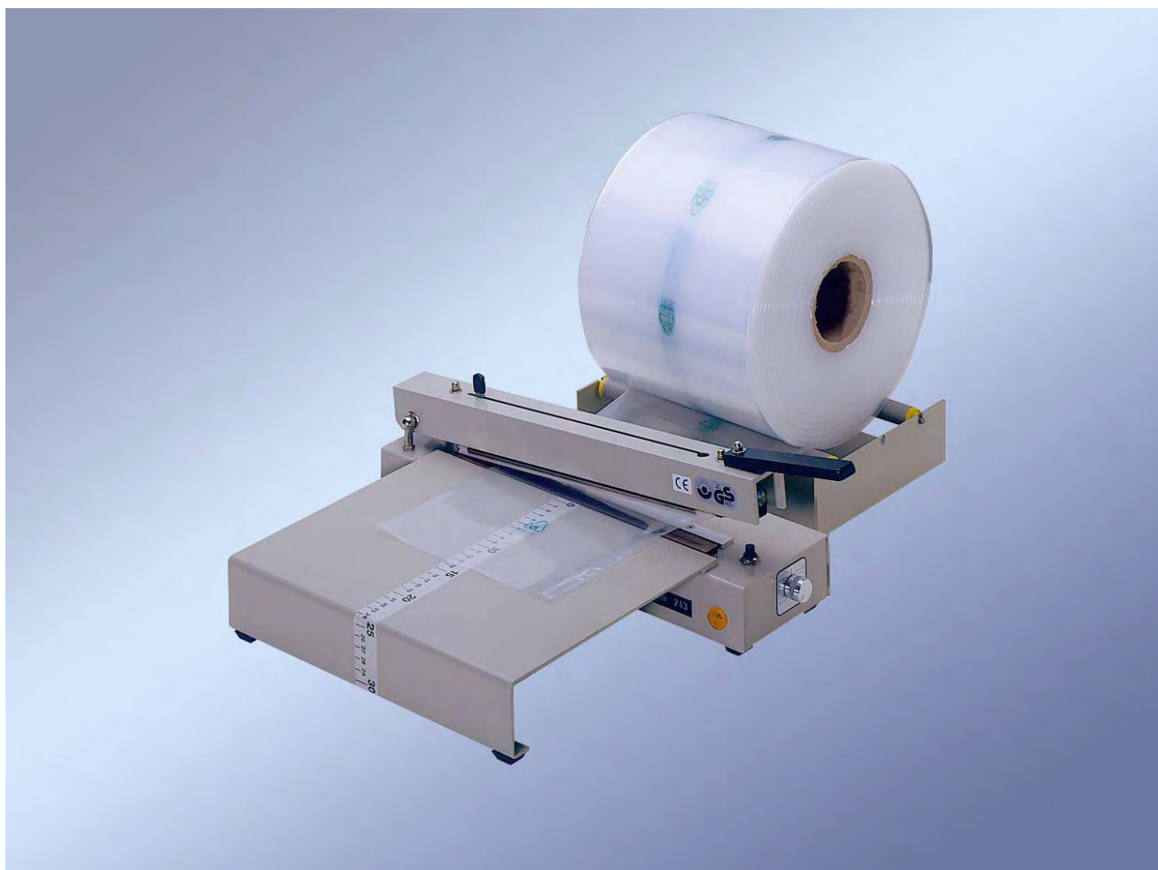
„polystar®“ 243 fóliavágóval (SV), munkaasztallal és fóliagörgő tartóval
