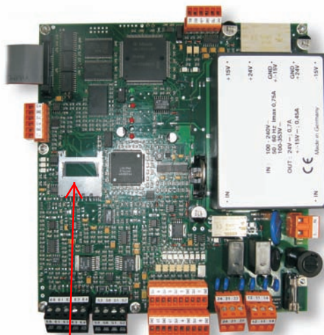
SD-MMC kártya aljzat
